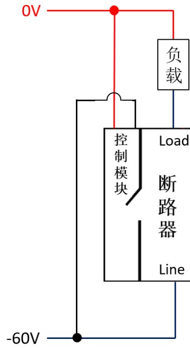
接线图
